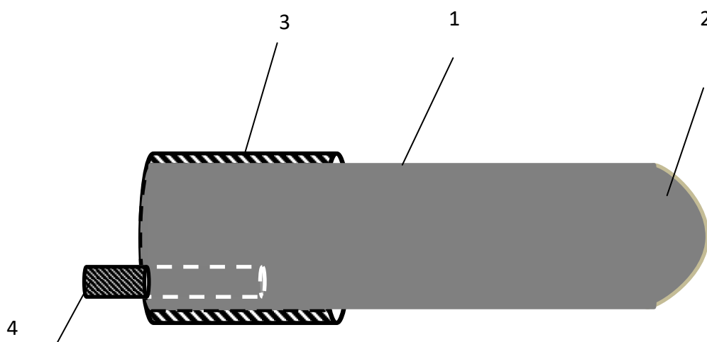
Рис. 2.6. Активний електрод: 1 – порожнистий циліндр; 2 – металічна півсфера; 3 – електроізоляційний матеріал; 4 – електричний контакт із гнучким ізольованим провідником.
